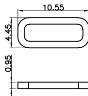
防水圈图示
